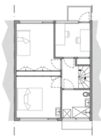
Eerste verdieping (nieuw)
