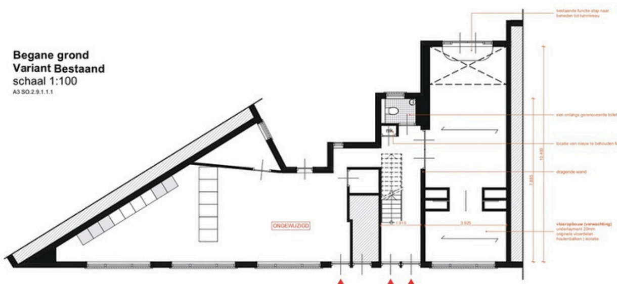
Begane grond Variant 02 schaal 1:100
