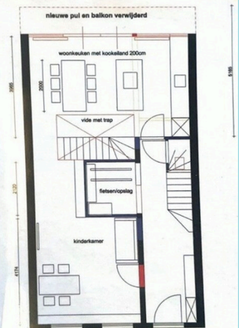
Voorstel 1 inrichting begane grond Verwijderen balkon, nieuwe pui en vide met 2e trap. Berging en fietsenstalling centraal in woning
