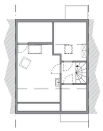
Tweede verdieping (nieuw)
