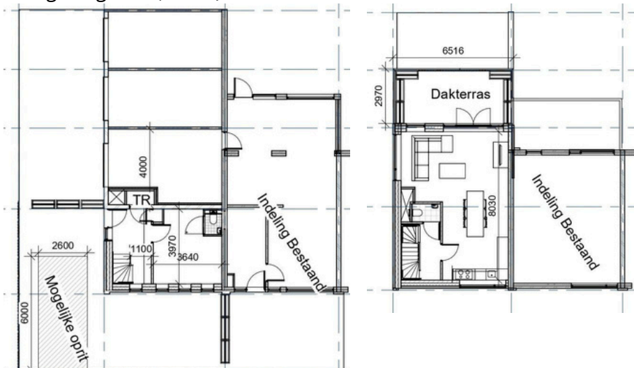
Eerste verdieping (nieuw)
